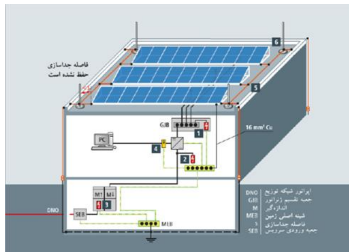
شکل شماره ۴: شیوه‌های همبندی سیستم اتصال زمین ۵ ( ساختمان با سیستم حفاظت خارجی و بدون فاصله جداسازی کافی )
